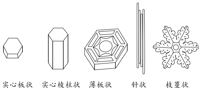
雪晶形态图
